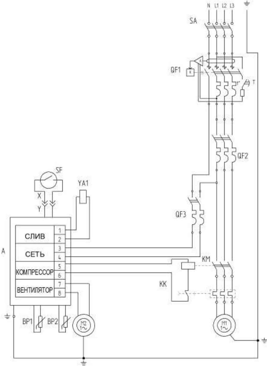
Рисунок 7 – Схема электрическая принципиальная для ОВ-1320М2.
