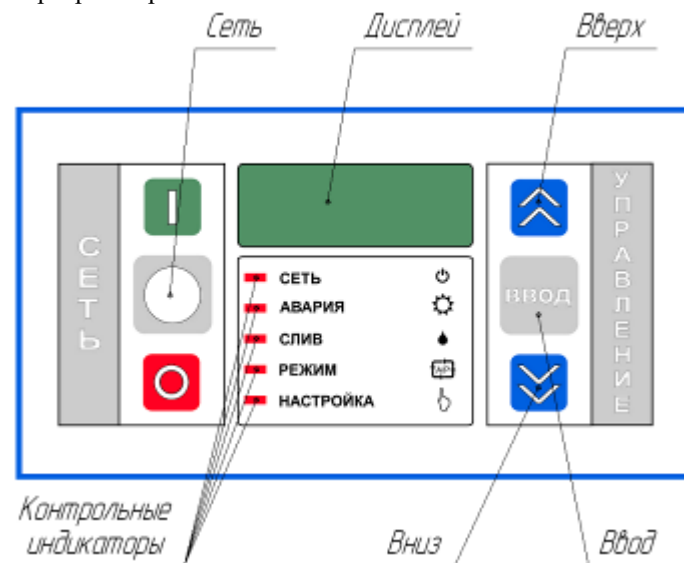
Рисунок 6 - Панель блока управления
