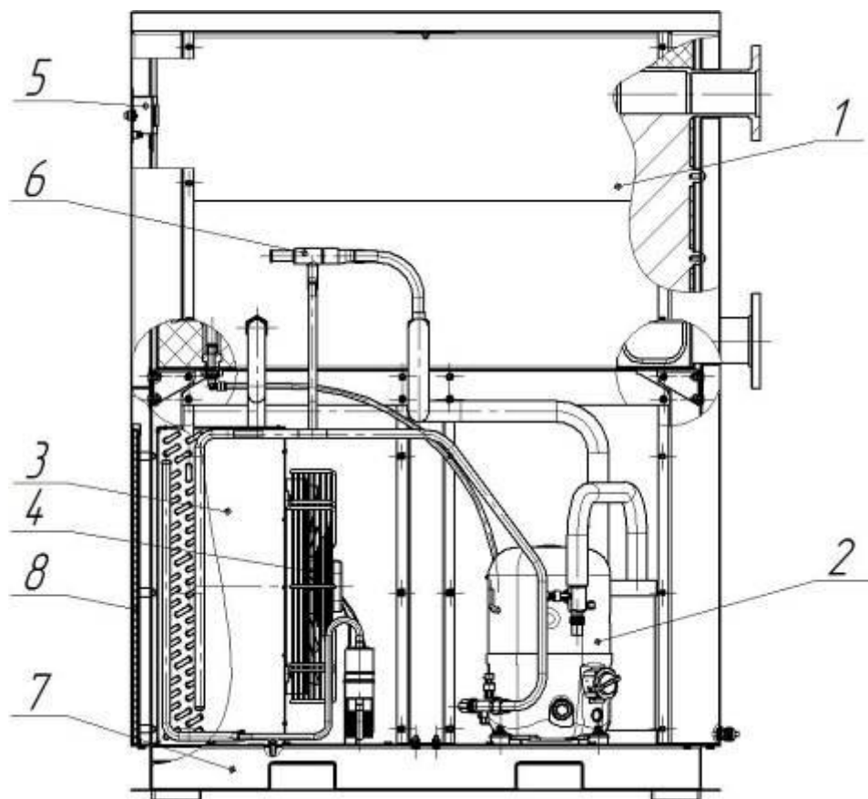
Рисунок 3 – Осушитель сжатого воздуха
